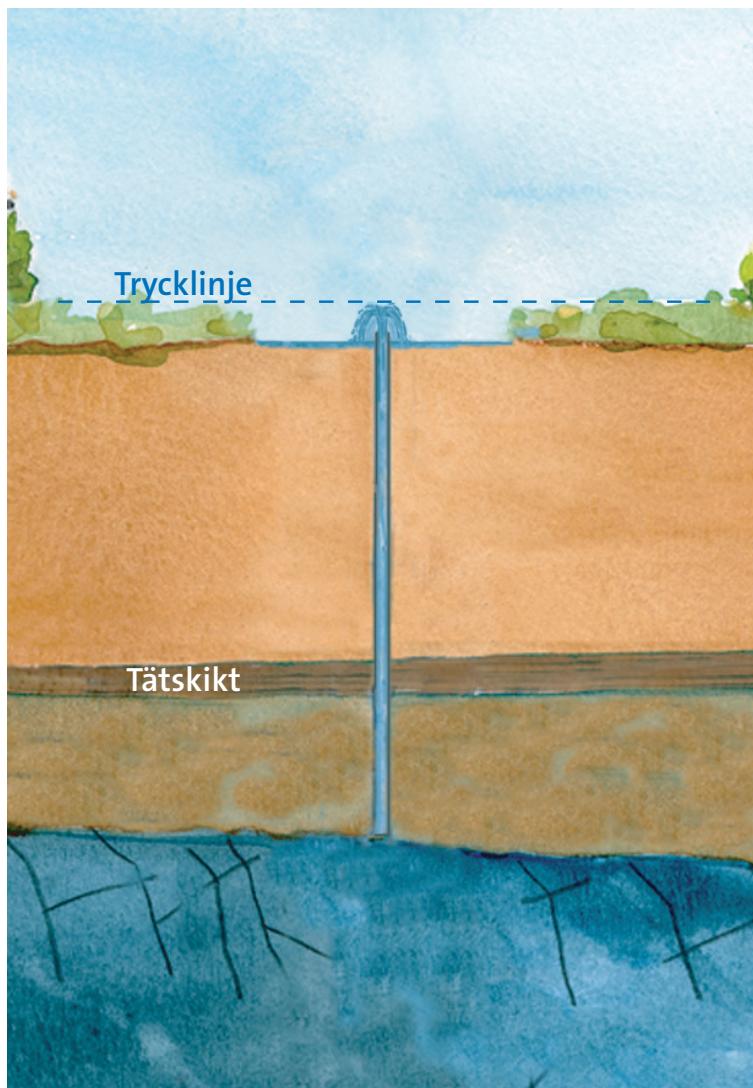
Figur 12. Artesiskt vatten. När en brunn borraras där vattnets trycknivå ligger över markytan, där marklagren utgörs av täta skikt, stiger vattnet. Då kan dränering eller avtätning av brunnen behövas.
