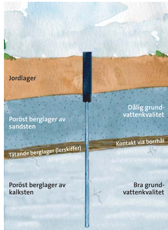
Figur 4. Olika sedimentära bergarter är ofta lagrade på varandra. Skifferar kan utgöra täta skikt mellan vattenförande lager så att vatten av god kvalitet inte blandas med sämre vatten.
